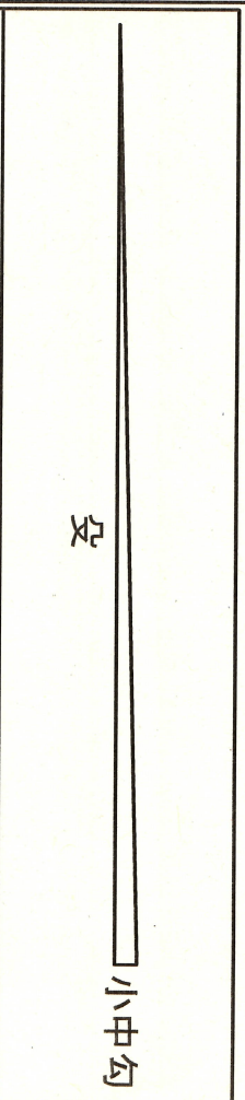
貫ほぞ孔上端・下端の勾配 (小中勾の返し勾配)
