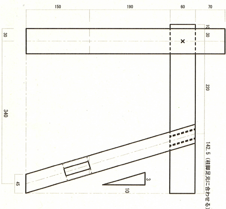
側面図
