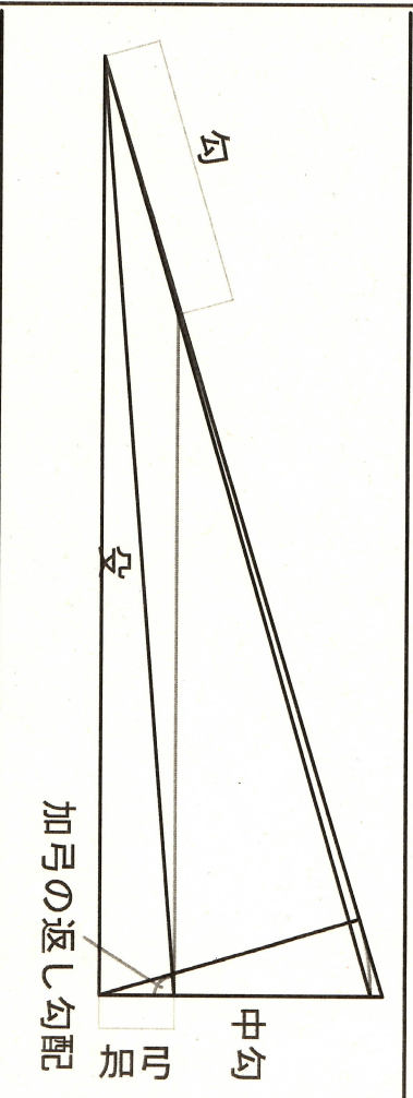
柱脚の癖 加弓勾配
