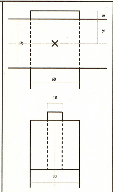
束柱・頭繋ぎ取り合い部詳細
